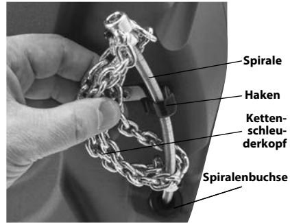
Abbildung 1C – Spiralenende/ Kettenschleuderkopf
