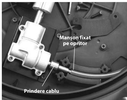
Figura 15 – Încuirea ansamblului cablului
