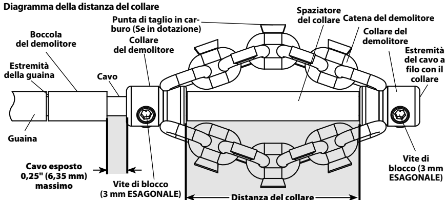
Figura 10 – Installazione/regolazione del Demolitore a catena
