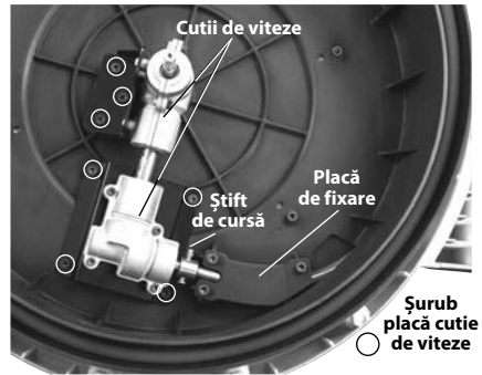
Figura 14 – carcasă mașină pentru curățarea scurgerilor deschisă
