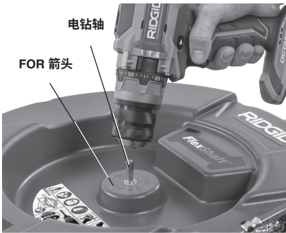
图 4 – 将电钻连接到电钻轴
