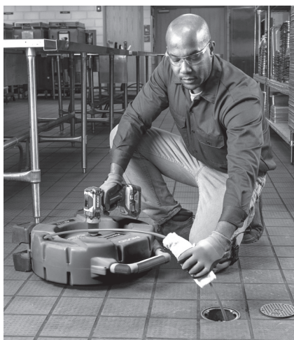
图 13 – 向钢索护套管涂抹润滑剂
