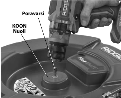
Kuva 4 – Pora-akselin kiinnittäminen pora-akseliin
