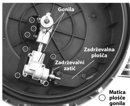
Slika 14 - Odprto ohišje naprave za čiščenje odtokov
