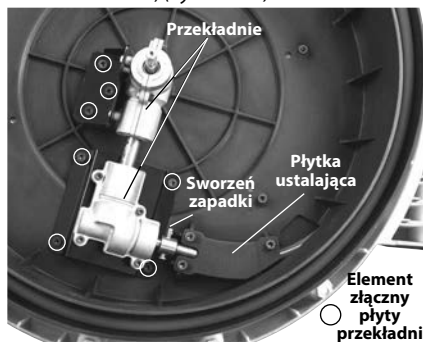
Rysunek 14 – Otwarta obudowa maszyny do przepychania odpływów
