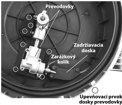
Obrázok 14 – Otvorené teleso zariadenia na čistenie odtokov
