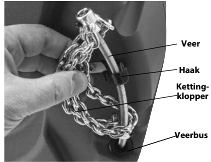
Figuur 1C – Veeruiteinde/kettingklopper
