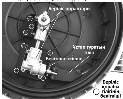
14-сурет — Ашылған ағын құбыры тазалағышының корпусы
