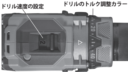
図6-ドリルの設定
