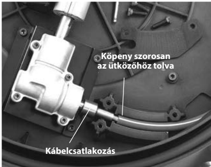
15. Ábra – A kábelszerelvény cseréje
