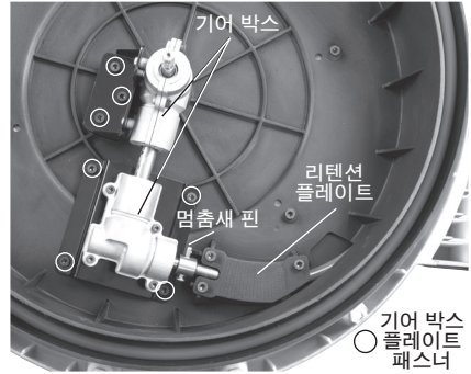
그림 14 - 열려 있는 드레인 클리너 하우징
