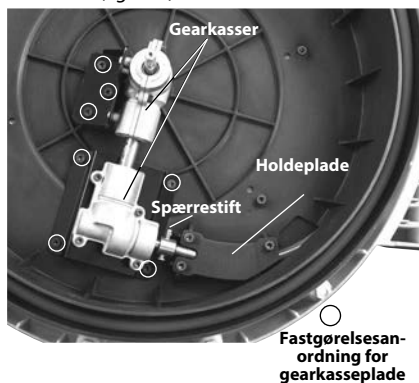
Figur 14 – Åbent afløbsrensemaskinehus
