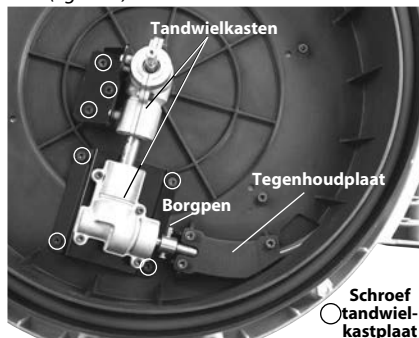
Figuur 14 – Geopende behuizing van de afvoertstopper
