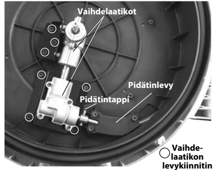
Kuva 14 – Viemärinavauslaitteen kotelo avattuna
