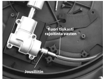
Kuva 15 – Jousikokoonpanon vaihtaminen
