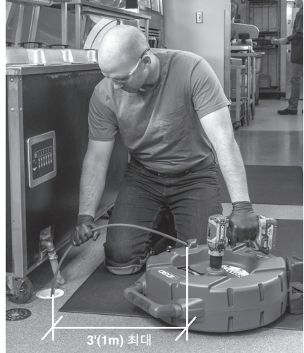
그림 11 - 작업 자세
