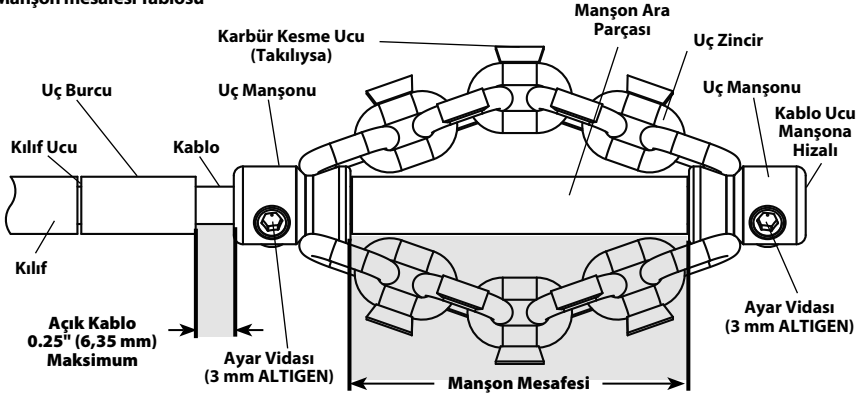
Şekil 10 – Zincirli Uç Takılması/Ayarlanması
