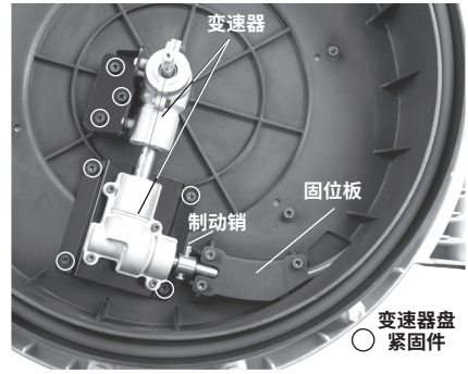
图 14- 管道疏通机壳体打开
