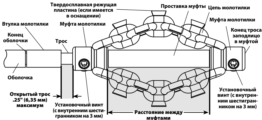
Рис. 10 - Установка/регулировка цепной молотилки
