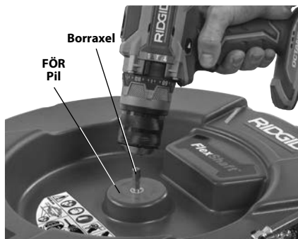
Figur 4 – Fästa borren på borraraxel
