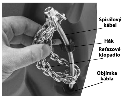
Obrázok 1C – Koniec kábla/retazové klopadlo
