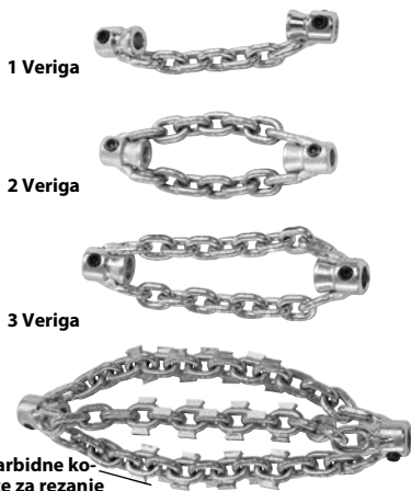
Slika 8 – Spiralna žagasta rezila
