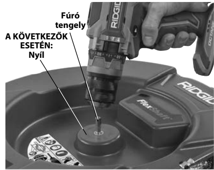
4. Ábra – A fűrógép csatlakoztatása a fűrtengelyhez
