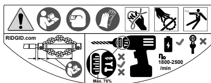
Obrázek 2 – Výstražný štítek
