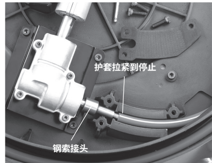
图 15 - 更换钢索组件
