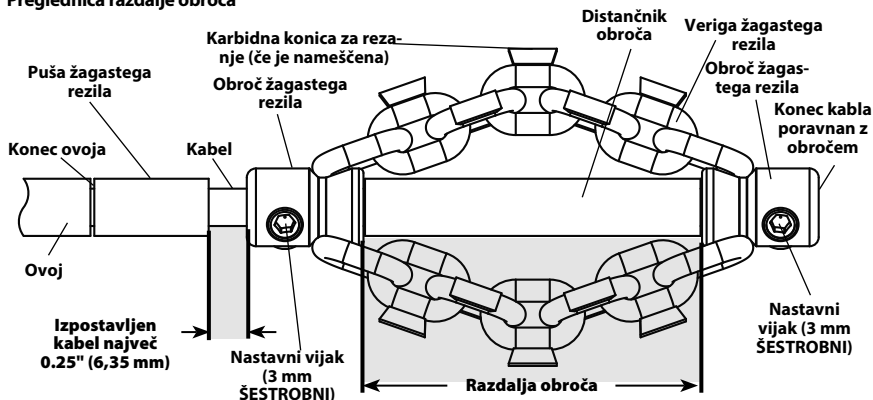
Slika 10 - Namestitvev/nastavljanje spiralnega žagastega rezila
