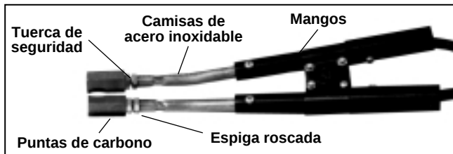
Figura 2b – Mangos y puntas de carbono de la RT-175
