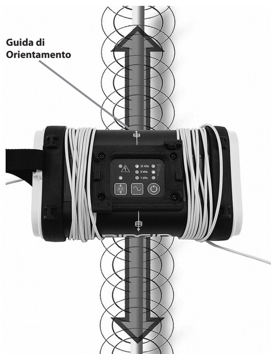
Figura 10: Orientamento rispetto alla linea – Modalità induttiva
