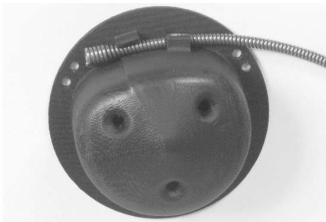
Figure 16 – Fixation du câble au tambour interne
