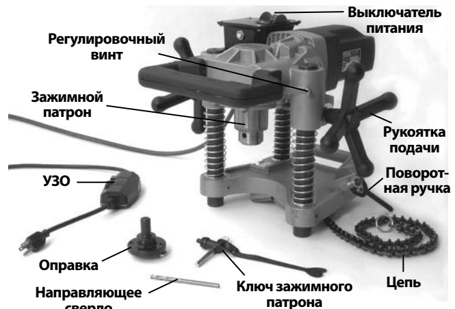
Рис. 1 – Модель HC-450 со стандартными принадлежностями
