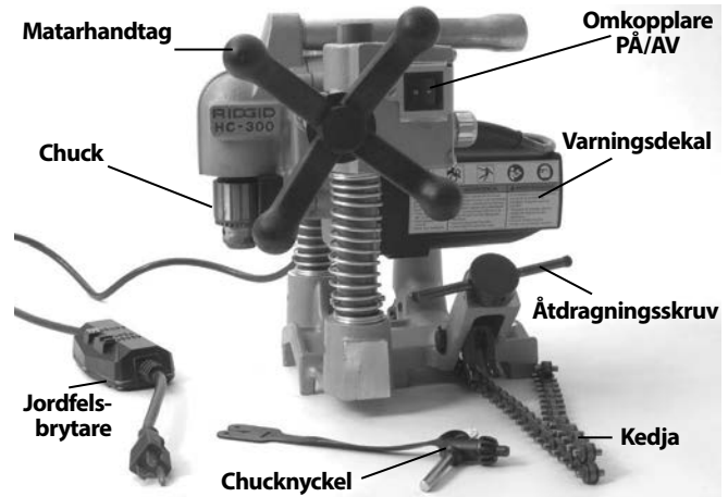
Figur 2 – HC-300 med standardutrustning
