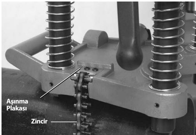
Şekil 5 – HC-450 Zincirinin Asılması
