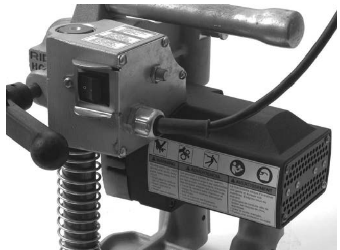
Figur 4B – HC-300-advarelsmærkater
