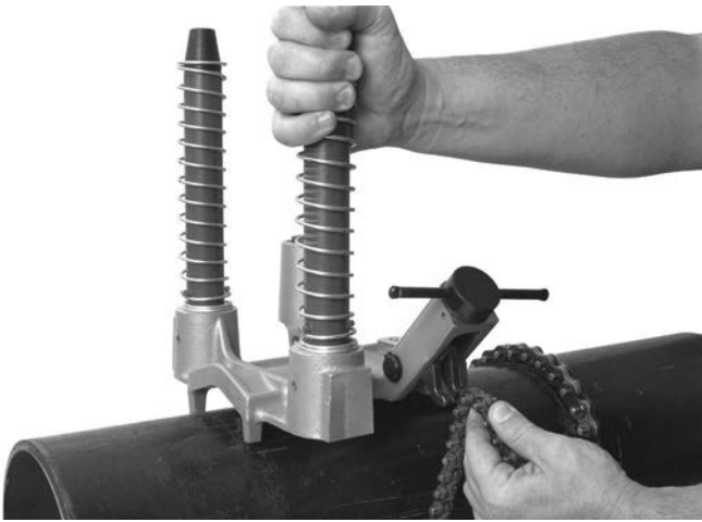
Figur 8 – Feste kjettingen
