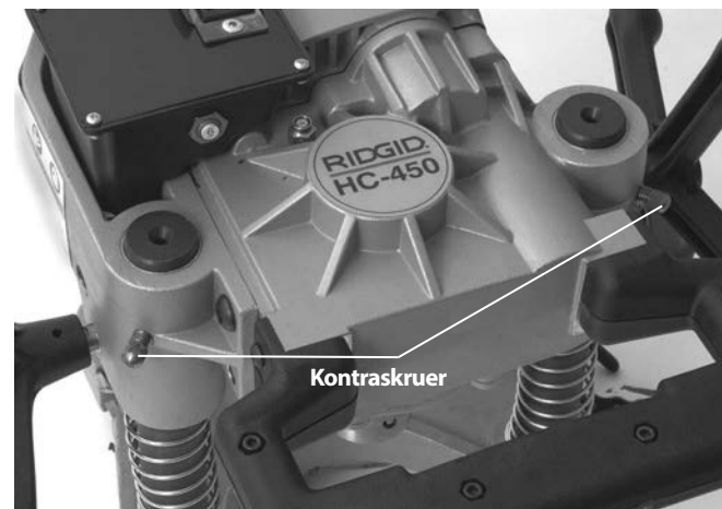
Figur 13 – Justering af kontraskruer
