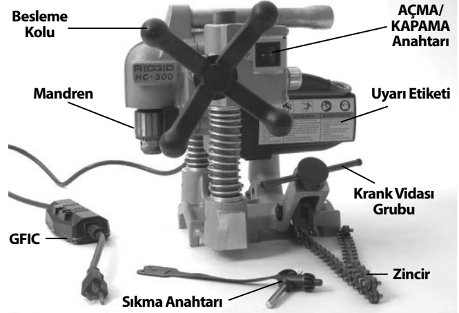
Şekil 2 – Model HC-300 Standart Ekipman ile
