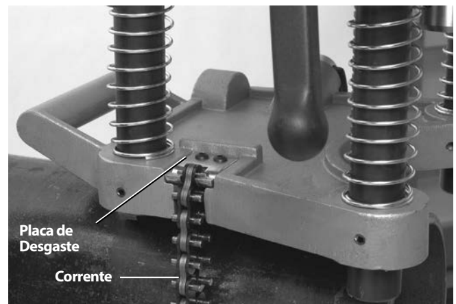
Figura 5 – Fixação da Corrente da HC-450
