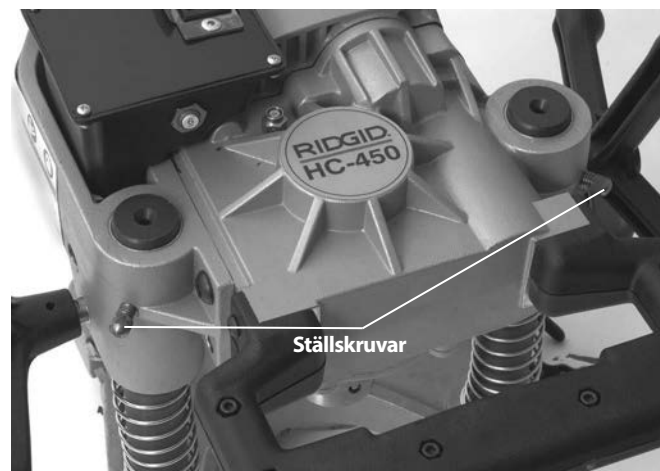
Figur 13 – Justera ställskruvarna
