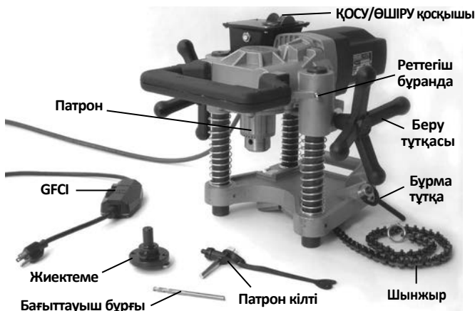
1-сурет – Стандартты жабдықпен HC-450
