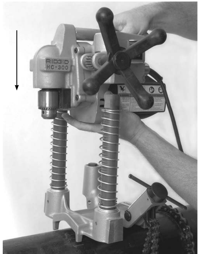
Slika 9 – Pritrditev sklopa motorja modela HC-300 na podstavek
