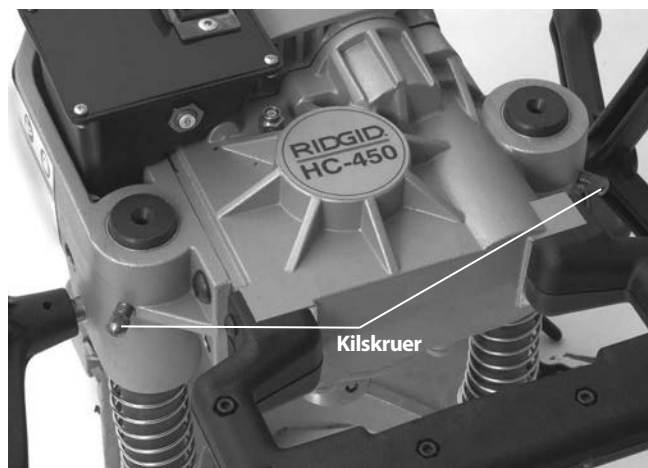
Figur 13 – Justere kilskruer
