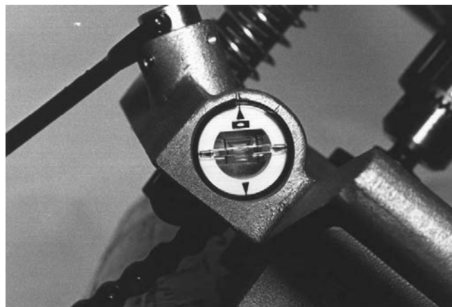
Slika 6 – Vodna tehtnica na električni kronska žagi HC-450
