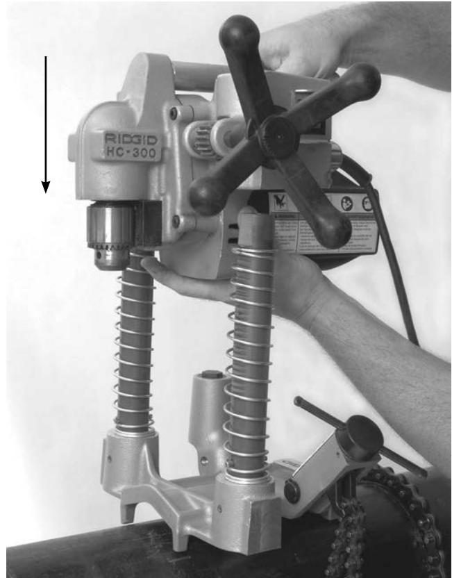
Figura 9 – Fixarea ansamblului motorului HC-300 la ansamblul bazei
