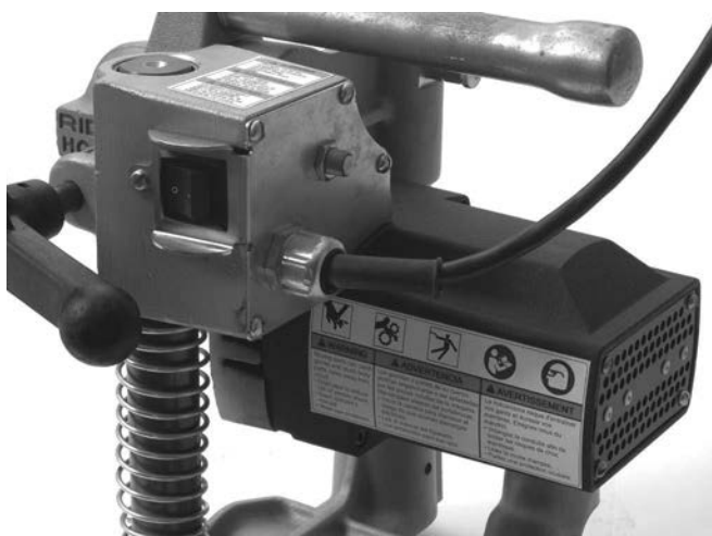
4B-сурет – HC-300 ескерту жапсырмалары
