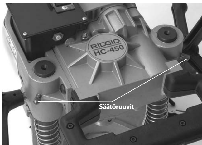
Kuva 13 – Säätöruuvien säätö
