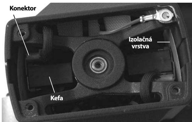
Obr. 12 – Umiestnenie kefy - Zložený kryt motora
