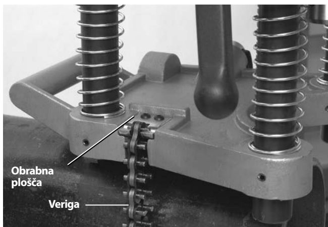
Slika 5 – Zatkanje verige HC-450
