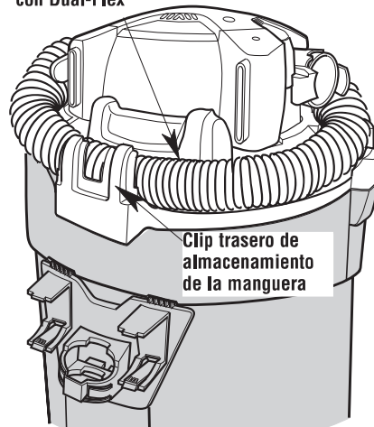
Manguera con fijación positiva Tug-A-Long con Dual-Flex
