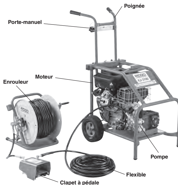
Figure 2 – Dégorgeoir haute-pression KJ-3100
