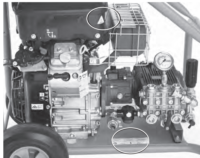
Figura 7 E – Etiquetas de advertencias en la KJ-3100
