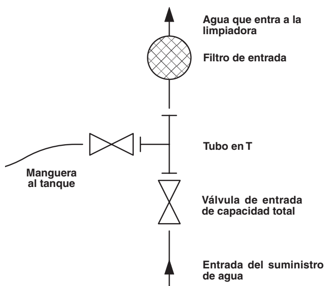
Figura 10 – Conexiones al emplear un tanque de agua como suministro
