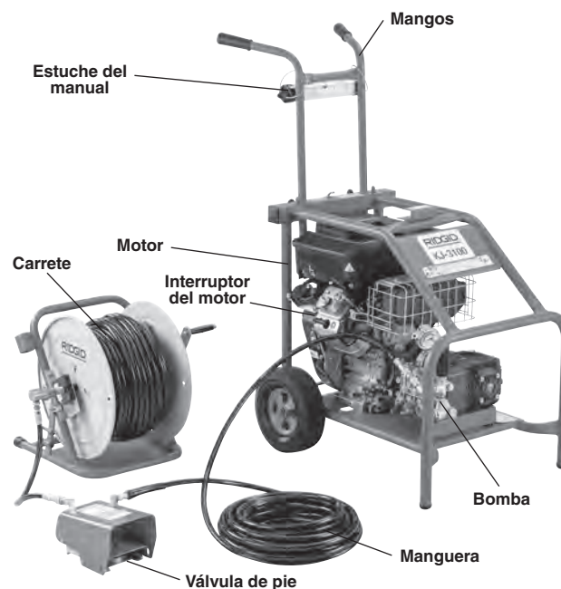
Figura 2 – Máquina limpiadora de agua a alta presión KJ-3100
