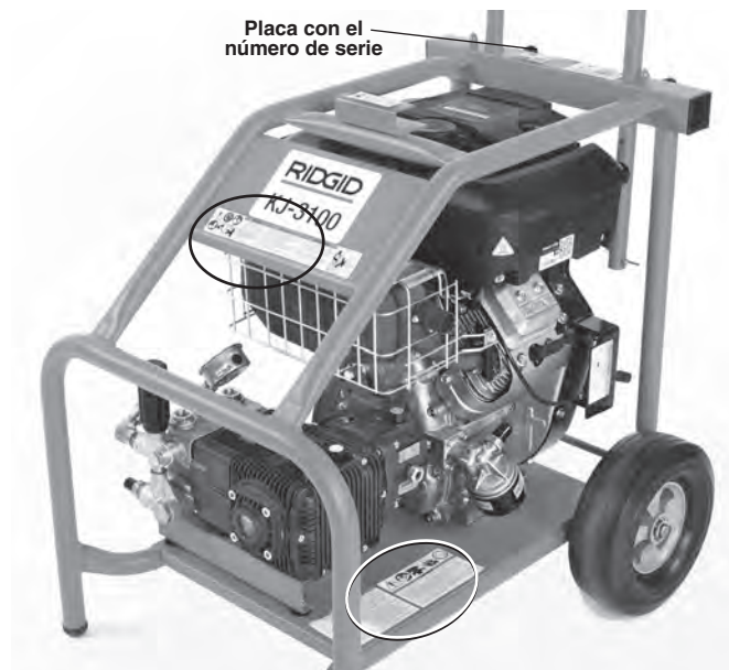
Figura 7 D – Etiquetas de advertencias en la KJ-3100
