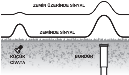
Şekil 6 – Manyetik Dedektörün Yerden Yükseltilmesi İstenmeyen Sinyalleri En Aza İndirir
