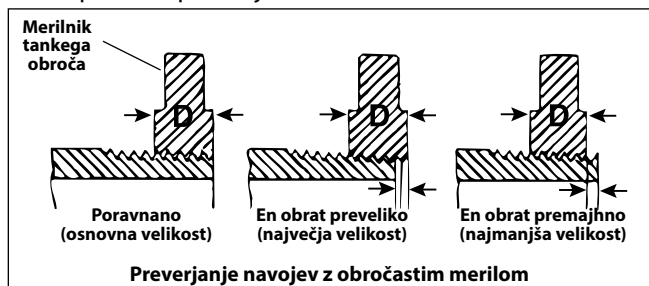
Slika 16 – Preverjanje velikosti navoja
