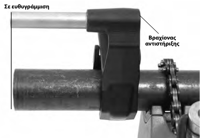
Εικόνα 10Α – Τοποθέτηση του βραχίονα αντιστήριξης
