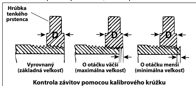
Obrázok 16 – Kontrola veľkosti závitov
