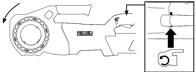
Рис. 5B - Положение переключателя РЕВЕРС (против часовой стрелки)
