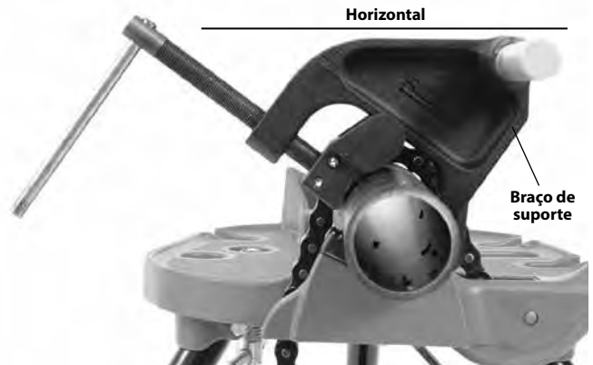
Figura 10A – Posicionamento do Braço de Suporte
