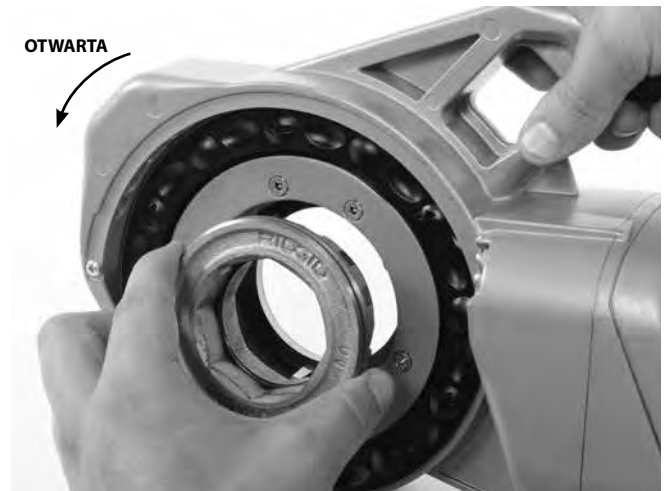
Rysunek 7 – Montaż adaptera
