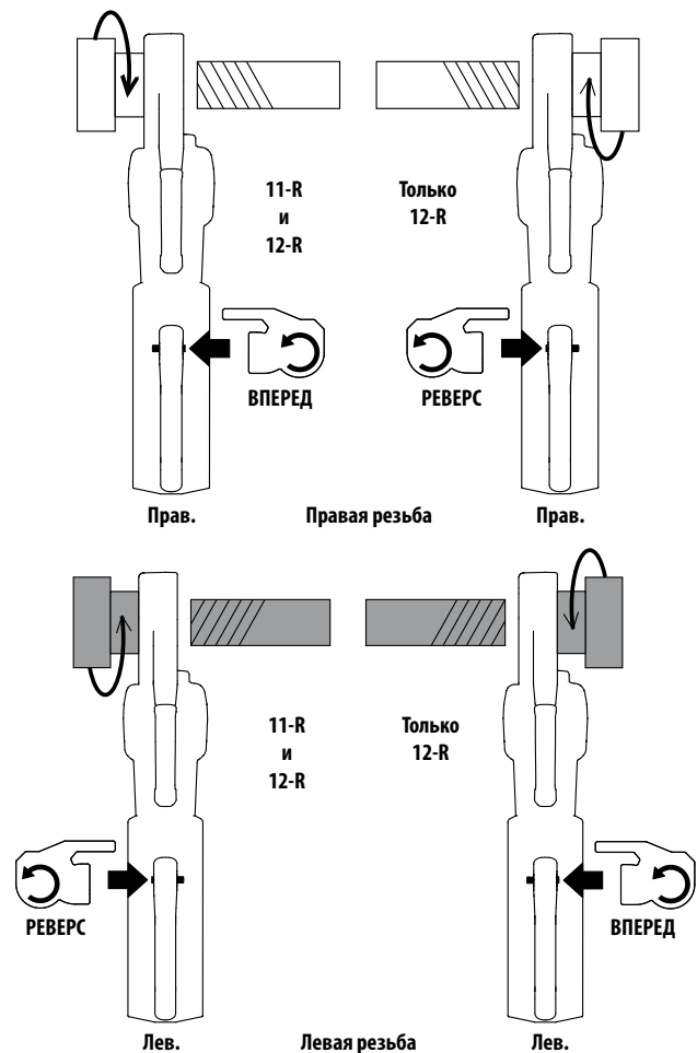
Рис. 9 - Ползунковый переключатель вперед/назад/ориентация резьбонарезной головки
