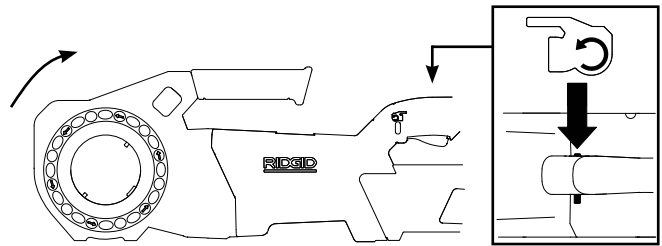
Рис. 5A - Положение переключателя ВПЕРЕД (по часовой стрелке)
