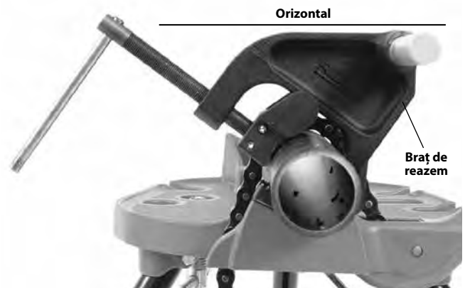
Figura 10A – Poziționarea brațului de reazem
