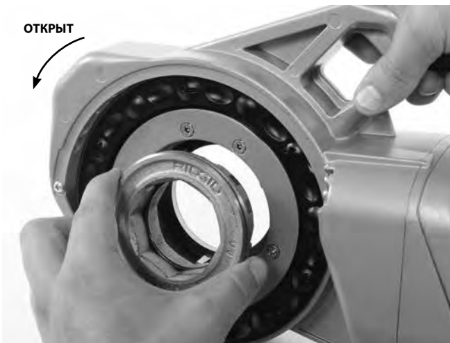
Рис. 7 – Установка переходника
