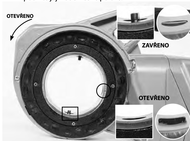
Obrázek 6A – Upínací mechanismus (760 FXP 12-R)
