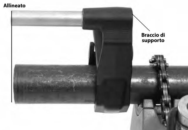
Figura 10B – Posizionamento del braccio di supporto
