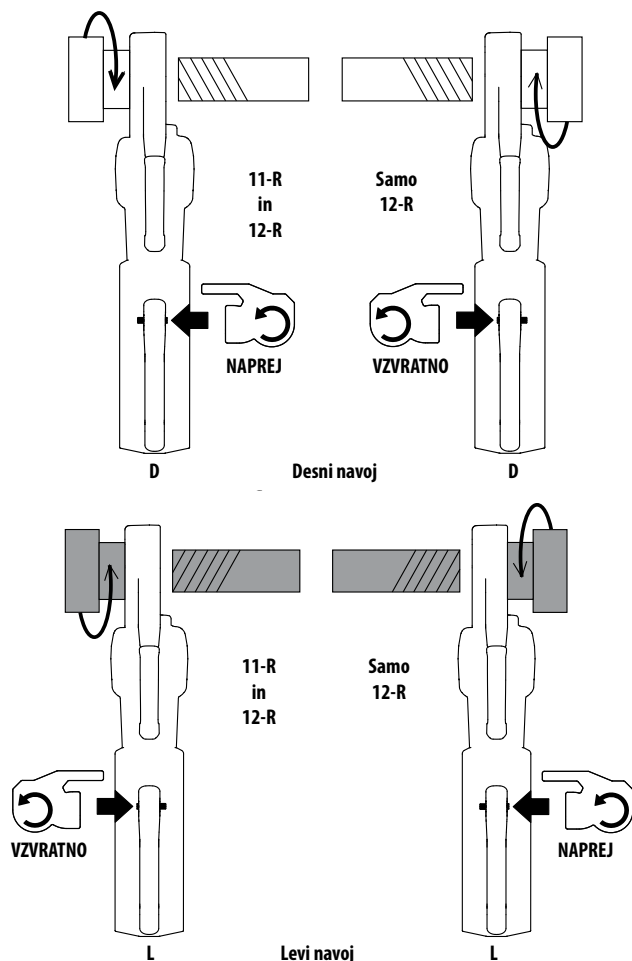
Slika 9 – Drсно stikalo naprej/nazaj/usmeritev glave navojnega rezalnika
