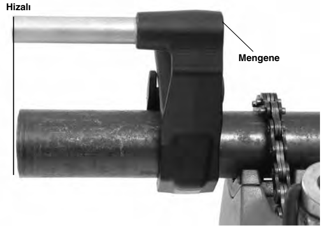
Şekil 10A – Destek Kolununun Konumlandırılması
