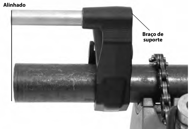
Figura 10A – Posicionamento do Braço de Suporte
