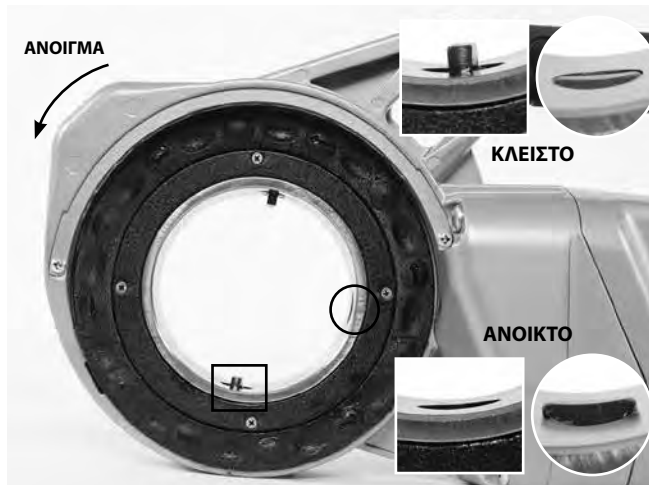
Εικόνα 6A – Μηχανισμός συγκράτησης (760 FXP 12-R)
