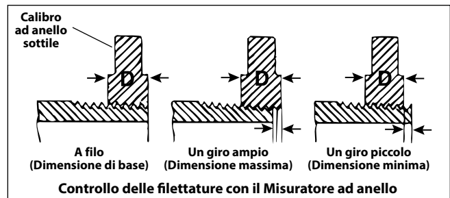
Figura 16 – Controllo della dimensione della filettatura
