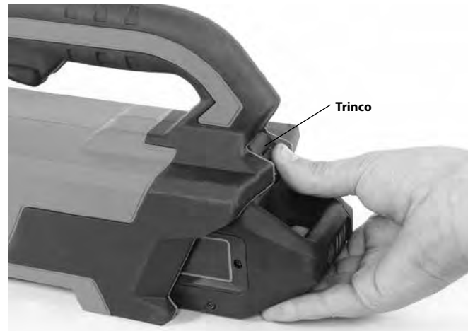
Figura 12 – Trinco da Bateria
