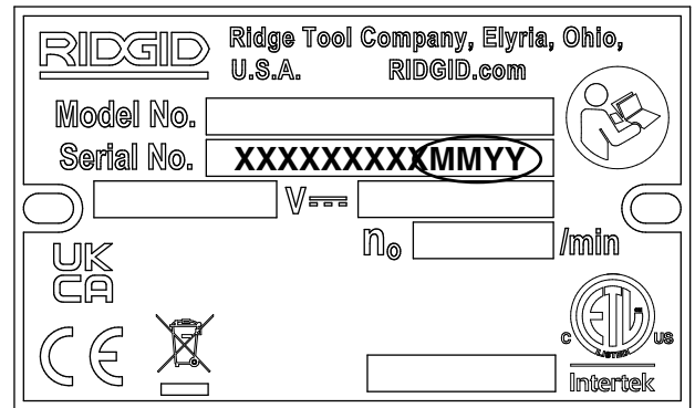
Figure 3 – Plaqué signalétique de l'appareil
