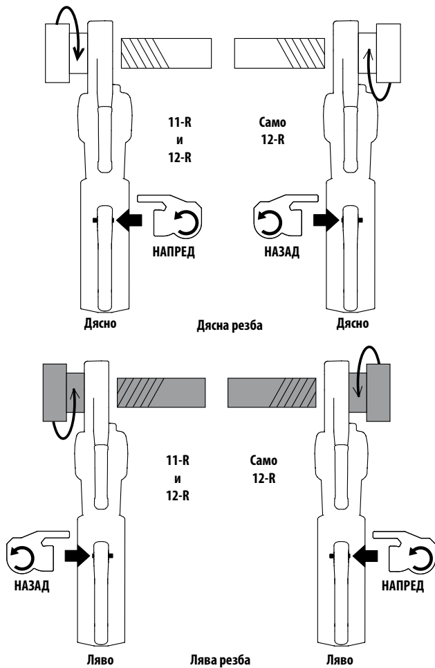
Фигура 9 – Ориентация на Плъзгащ превключвател Напред/Назад / Глава за матрици
