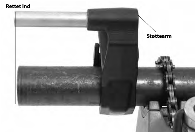
Figur 10B – Placering af støttearmen
