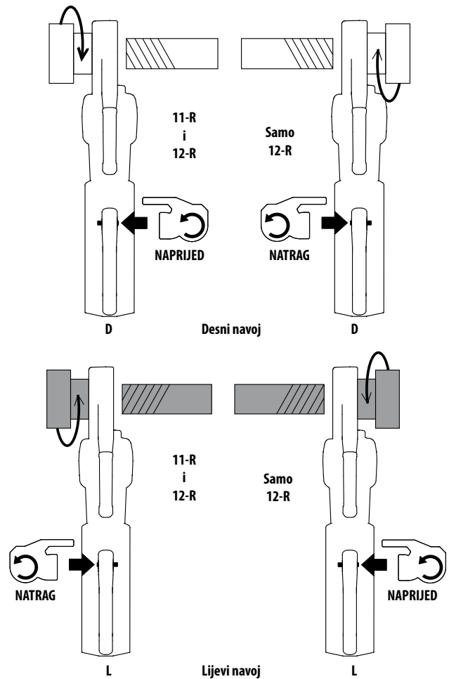
Slika 9 – Usmjerenje klizne sklopke za naprijed/natrag i narezne glave
