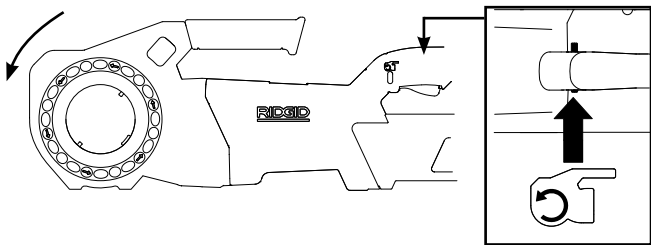
Obrázok 5B – Poloha prepínača DOZADU (proti smeru hodinových ručičiek)
