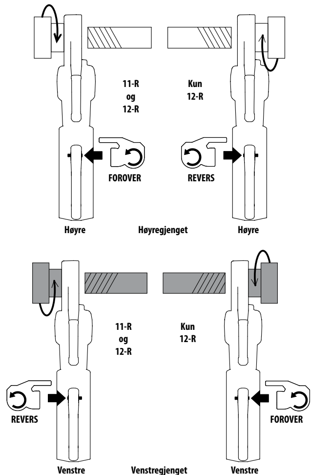
Figur 9 – Forover/Revers-glidebryter/Gjengehode-retning
