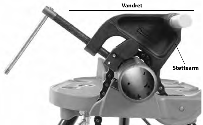
Figur 10A – Placering af støttearmen
