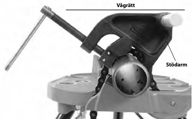
Figur 10A – Placera stödarmen
