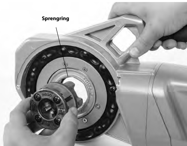
Figur 8 – Montering av 1¼" eller mindre 11-R gjengehoder (bare 760 FXP 11-R)
