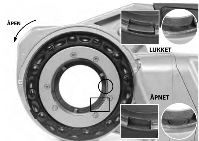
Figur 6B – Festemekanisme (760 FXP 11-R)
