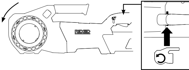
Figura 5B – Posição do Interruptor PARA TRÁS (Para a Esquerda)
