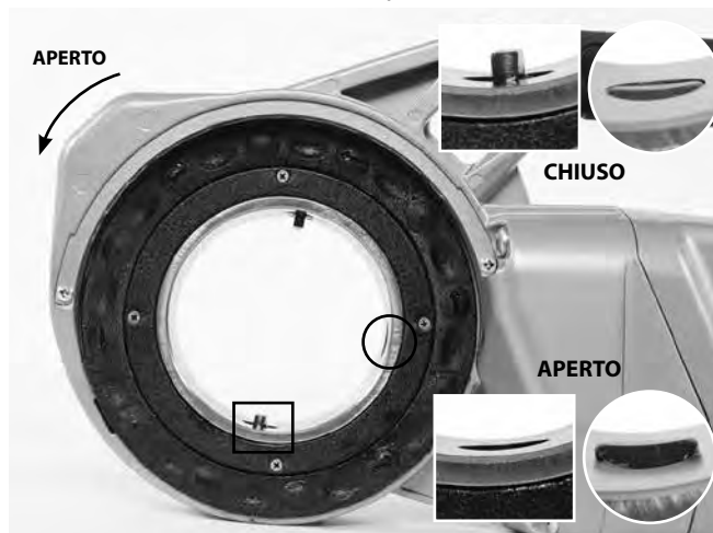
Figura 6A – Meccanismo di ritengo (760 FXP 12-R)
