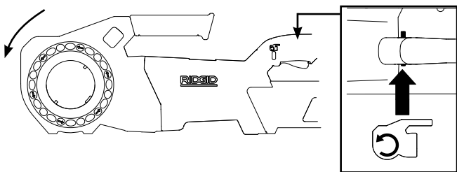
Obrázek 5B – Poloha spínače VZAD (proti směru hodinových ručiček)
