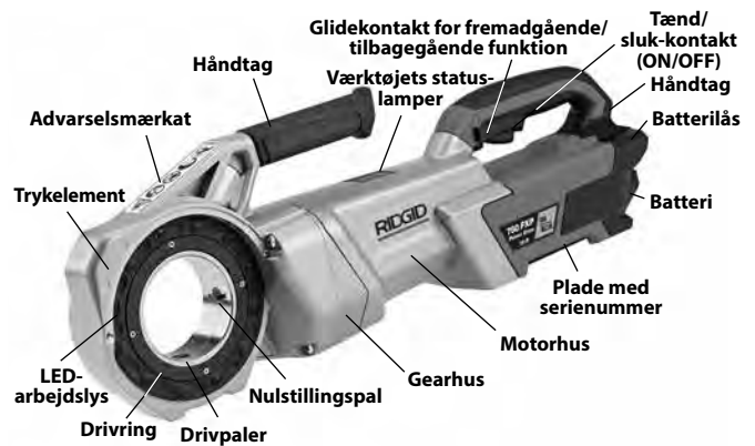
Figur 1 – Elektrisk rørdrev 760 FXP
