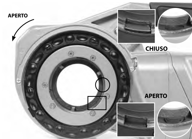
Figura 6B – Meccanismo di ritengo (760 FXP 11-R)
