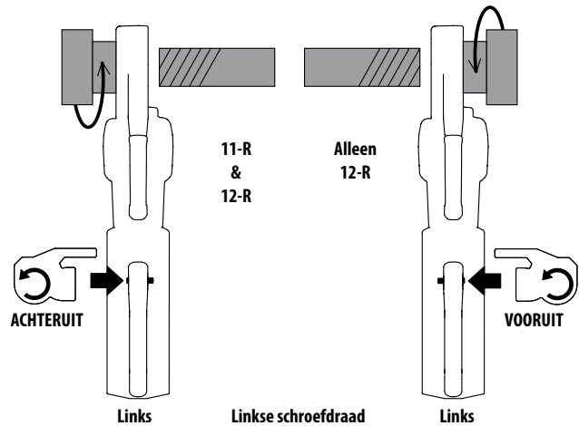
Afbeelding 9 – Richting van schuifschakelaar voor vooruit/achteruit - draadsnijkop
