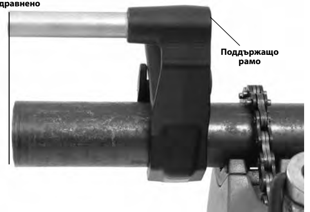
Фигура 10A – Позициониране на поддържащо рамо Подравнено
