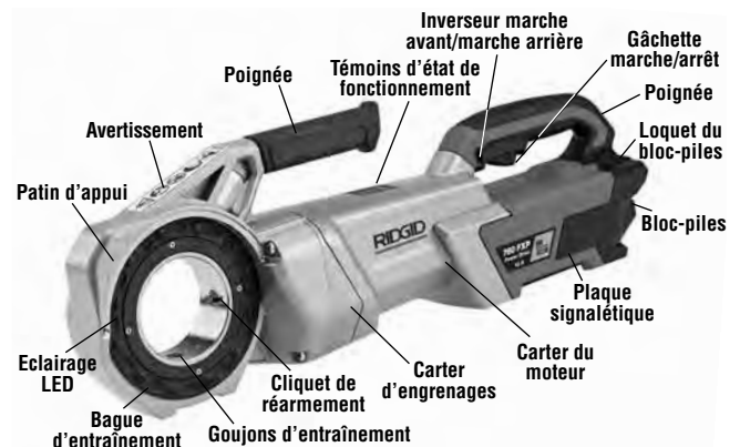
Figure 1 – Système d'entraînement 760 FXP Power Drive
