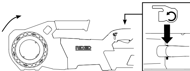
Rysunek 5A – Położenie przełącznika odpowiadające obrotom przednim (zgodnie z ruchem wskazówek zegara)
