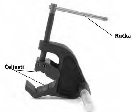
Slika 2 – 692 Potporna stega
