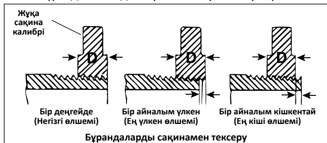
16-сурет – Бұранда өлшемін тексеру
