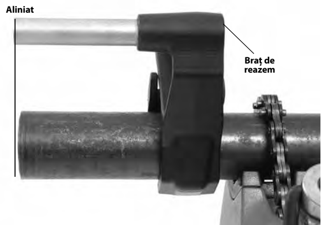
Figura 10A – Poziționarea brațului de reazem
