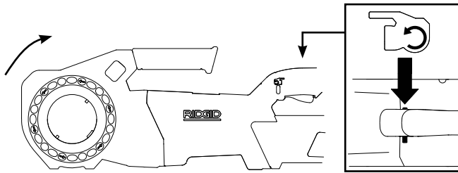
Figura 5A – Posição do Interruptor PARA A FRENTE (Para a Direita)
