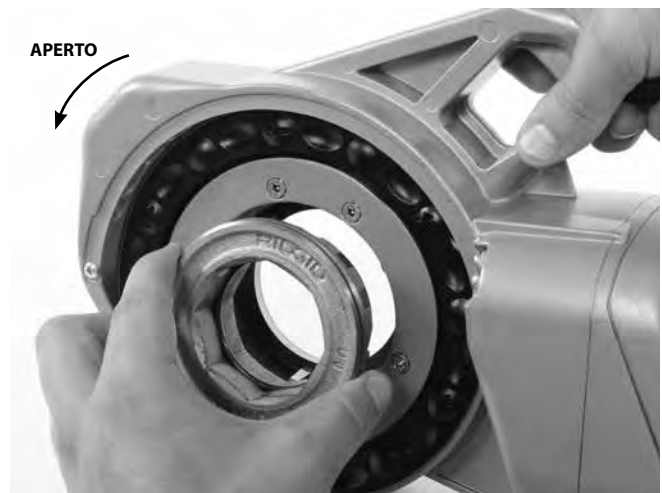
Figura 7 – Installazione adattatore
