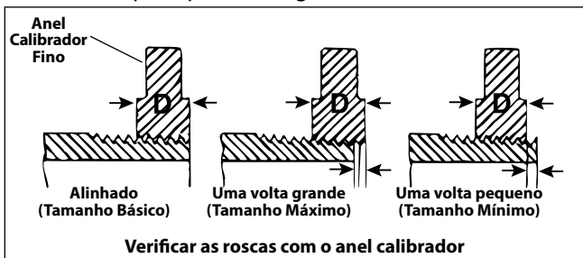
Figura 16 – Verificar o tamanho da rosca
