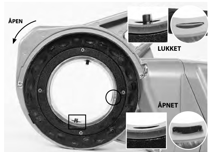
Figur 6A – Festemekanisme (760 FXP 12-R)
