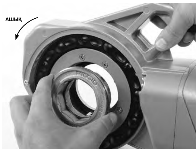
7-сурет – Жалғағышты орнату
