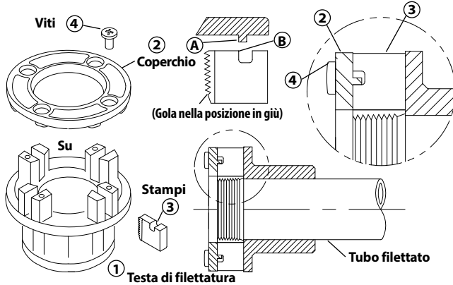
Figura 17 – Installazione degli Stampi nella Testa di filettatura
