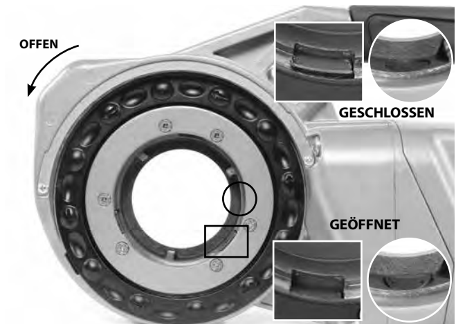
Abbildung 6B - Haltemechanismus (760 FXP 11-R)
