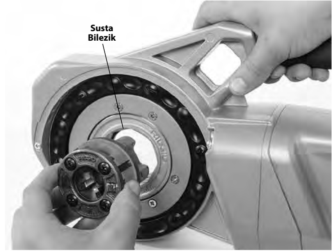
Şekil 8 – 1¼" veya Daha Küçük 11-R Pafta Kafalarının (yalnızca 760 FXP 11-R) takılması
