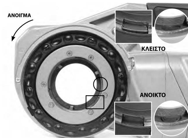
Εικόνα 6B – Μηχανισμός συγκράτησης (760 FXP 11-R)
