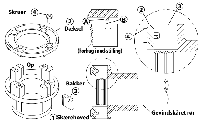
Figur 17 – Montering af bakker i skærehoved
