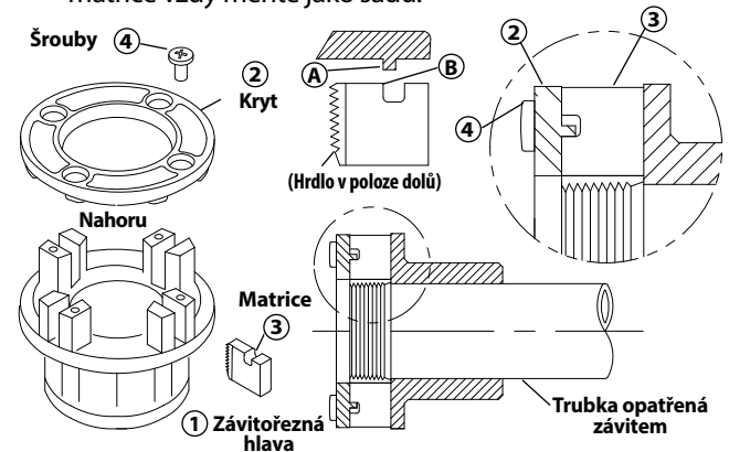
Obrázek 17 – instalace řezných matic do závitorežné hlavy
