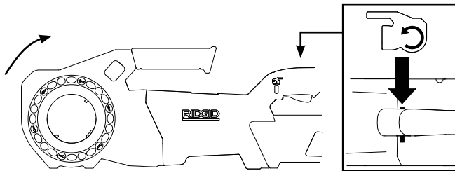
Figur 5A – FRAMÅT (medurs) omkopplarpöosition
