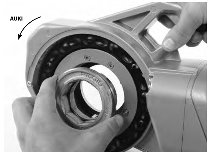
Kuva 7 – Sovittimen asennus
