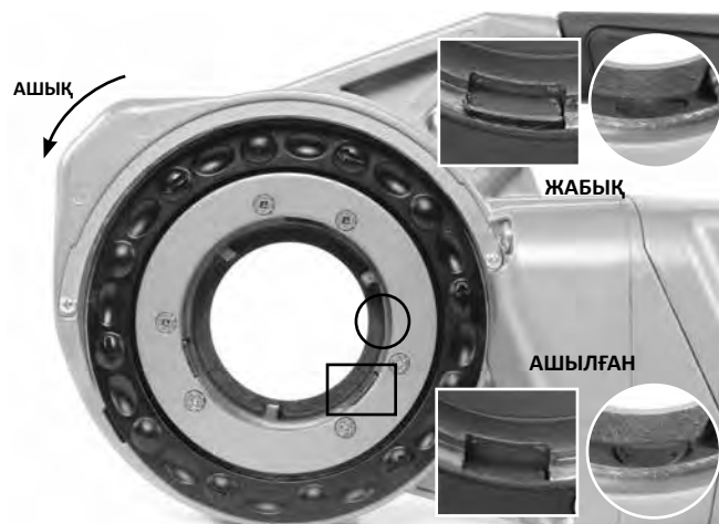
6B суреті – Ұстап тұру тетігі (760 FXR 11-R)
