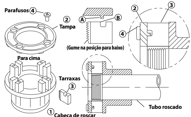
Figura 17 – Instalar tarraxas na cabeça de rosca
