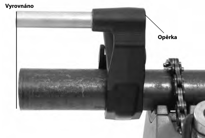
Obrázek 10A – Umístění opěrky
