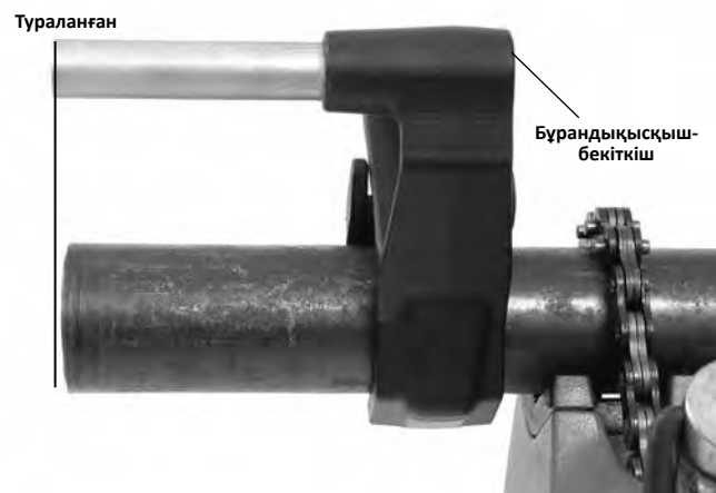
10B суреті – Бұрандама қысқышын орналастыру
