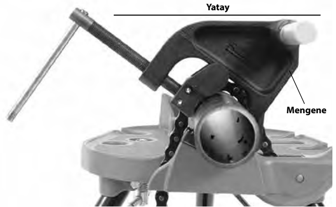
Şekil 10A – Destek Kolununun Konumlandırılması
