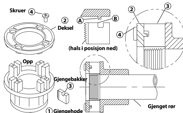
Figur 17 – Installere gjengebakker i gjengehodet
