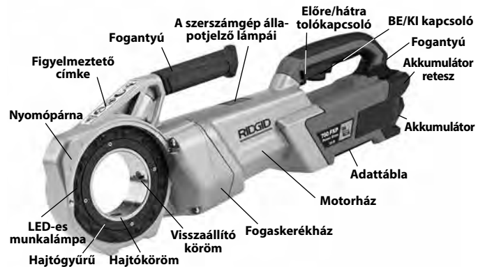
1. ábra – 760 FXP motoros hajtóegység
