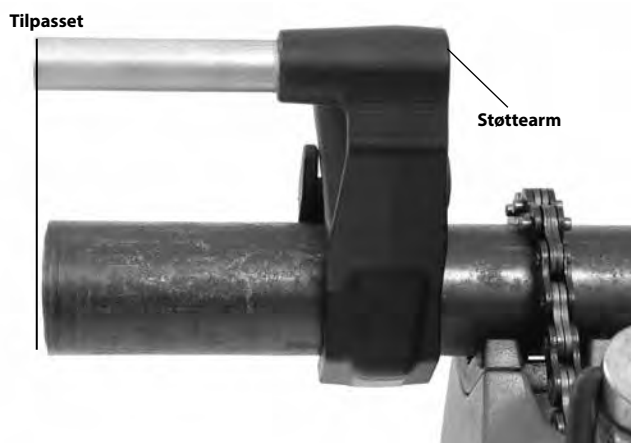
Figur 10A – Plassering av støttearmen
