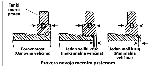
Slika 16 – Provera veličine navoja
