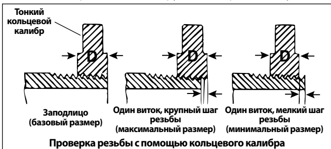
Рис. 16 – Проверка размера резьбы
