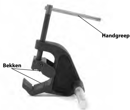
Afbeelding 2 – 692 Steunarm
