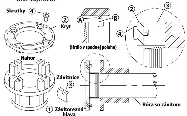
Obrázok 17 – Inštalácia závitnic do závitoreznej hlavy
