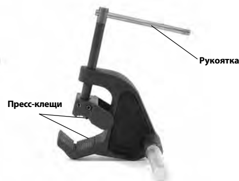
Рис. 2 - Струбцина-фиксатор 692
