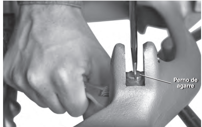
Figura 13 – Ajuste del perno de agarre
