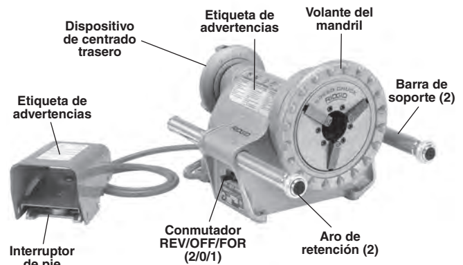
Figura 1 – Accionamiento motorizado Modelo 300
