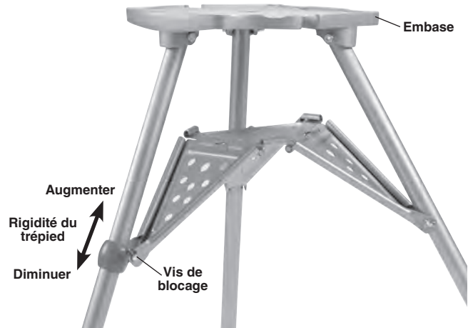
Figure 5 – Réglage du support de tablette
