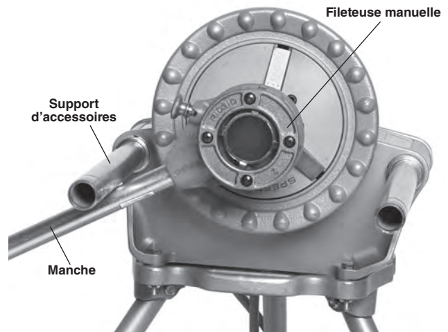
Figure 20 – Retrait de la tête de filière du tuyau fileté (Manche appuyé contre la sous-face du support)
