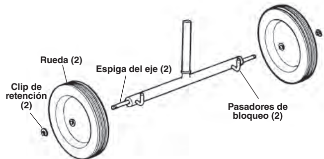
Figura 27 – Montaje del transportador No. 32
