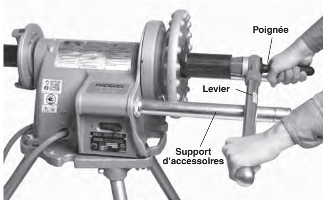
Figure 16 – Alésage des tuyaux à l'aide d'un alésoir manuel. (Gardez le levier de l'alésoir appuyé contre le support)
