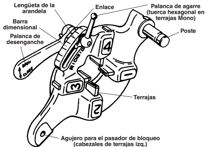
Figura 9 - Cabezal de terrajas de apertura rápida
