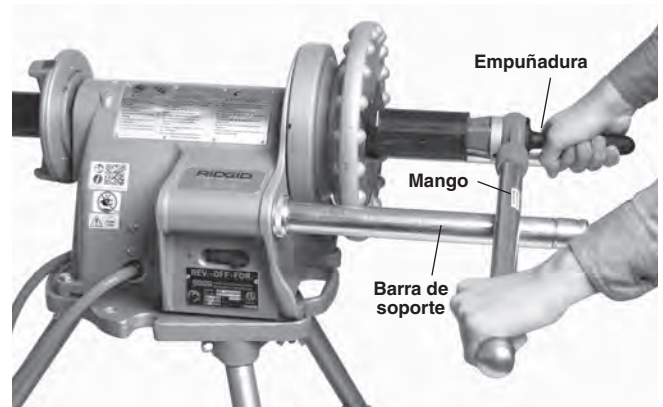
Figura 16 – Escariado de un tubo con un escariador manual. El mango del escariador debe mantenerse en contacto con la barra de soporte.
