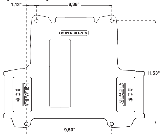
Figure 6 – Gabarit des trous d'embase du 300 Power Drive
