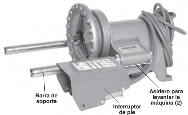
Figura 26 – La máquina sola, preparada para su transporte
