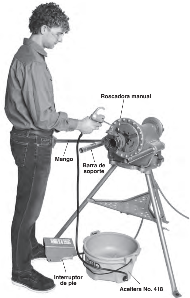
Figura 18 – Posición de trabajo correcta para roscar con roscadoras manuales; mantenga el mango de la roscadora en contacto con la barra de soporte.
