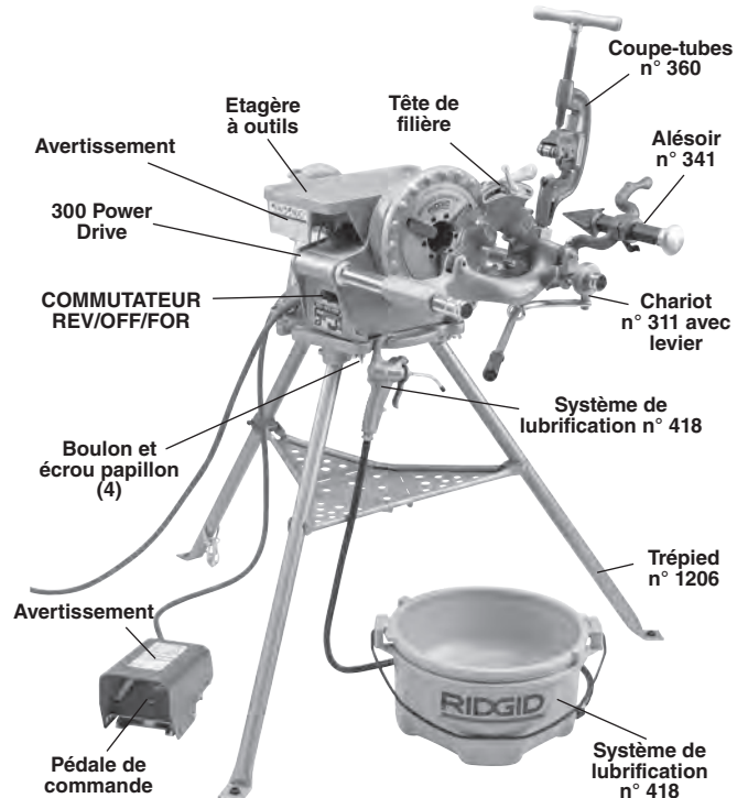
Figure 2 – Système d'entraînement 300 Power Drive Complete
