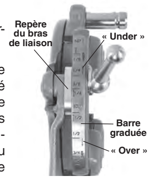
Figure 12 – Réglage du filetage
