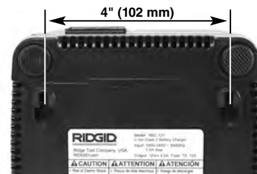
Figure 3 – Emplacement de l'avertissement apposé sur le chargeur
