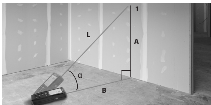
Figura 11 – Distanza orizzontale e verticale indiretta
