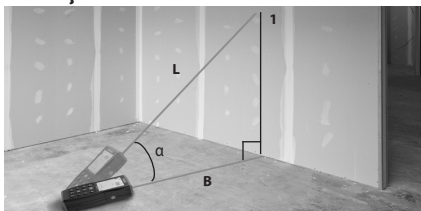
Figura 12 – Distanță orizontală indirectă
