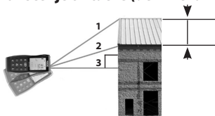
Slika 10 – Indirektno merenje korišćenjem tri tačke (delimična visina)
