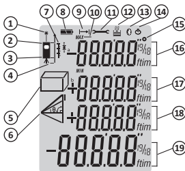
3-сурет — micro LM-400 лазерлік қашықтық өлшегішінің басқару тетіктері
