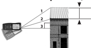
Рисунок 10 –Косвенное измерение между тремя точками (частичная высота)
