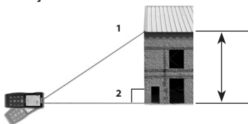
Figura 8 – Medição Indirecta Utilizando Dois Pontos
