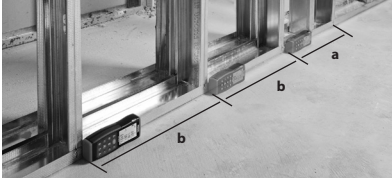
Şekil 16 - Belirleme Ölçümü
