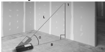
Figur 12 – Indirekt vågrät sträcka
