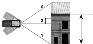
Obrázok 9 – Nepriame meranie pomocou troch bodov (celková výška)
