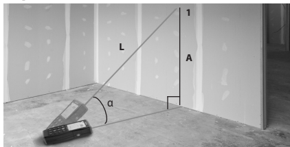
Obrázek 13 – Nepřímá vertikální vzdálenost
