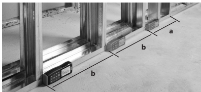
Kuva 16 – Paalutusmittaus
