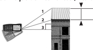
Figura 10 – Medição Indirecta Utilizando Três Pontos (Altura Parcial)
