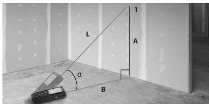
Figur 11 – Indirekt vågrätt och lodrätt avstånd
