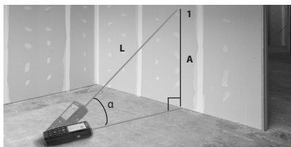
Figura 13 - Distanza verticale indiretta
