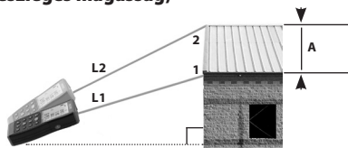
15. ábra – Közvetett mérés két ponttal (részleges magasság)
