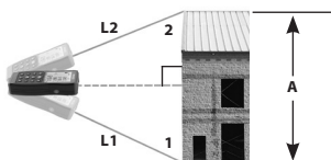
Figura 14 – Distanță verticală indirectă utilizând două puncte (înălțime totală)
