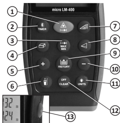
3-сурет — micro LM-400 лазерлік қашықтық өлшегішінің басқару тетіктері
