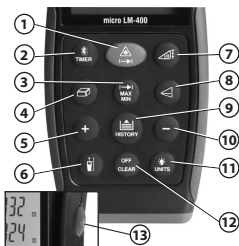
Kuva 3 – micro LM-400 Laseretäisyysmittari
