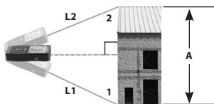
Figur 14 – Indirekt lodrät sträcka med två punkter (totalhöjd)
