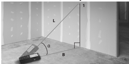
Slika 12 – Neizravna vodoravna udaljenost
