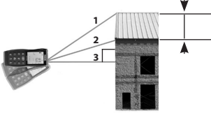
Şekil 10 – Üç Nokta Kullanarak Dolaylı Ölçüm (Kısmi Yükseklik)
