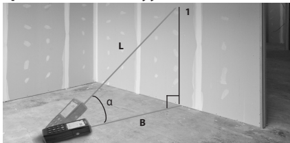
Kuva 12 – Epäsuora vaakaetäisyys
