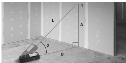
Figur 11 – Indirekte horisontal og vertikal afstand
