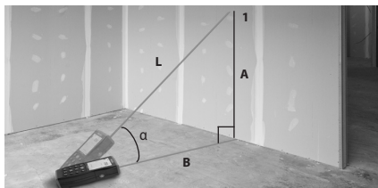
Obrázek 11 – Nepřímá horizontální a vertikální vzdálenost
