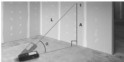
Figur 13 – Indirekte vertikal avstand
