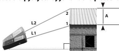
Kuva 15 – Epäsuora pystyettäisyys kahdella pisteellä (osakorkeus)
