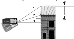
Figura 10 – Misurazione indiretta usando tre punti (Altezza parziale)
