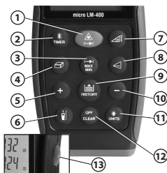
Obrázok 3 – Laserový merač vzdialenosti micro LM-400
