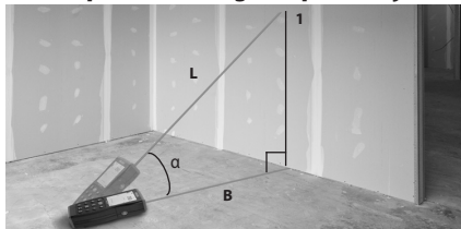
Rys. 12 – Pomiar pośredni odległości poziomej
