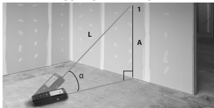
13. ábra – Közvetett függőleges távolság
