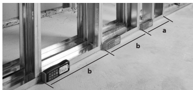
Obrázek 16 – Vytyčovací měření
