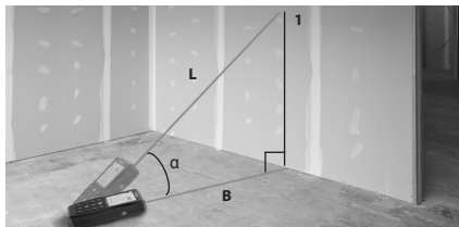
Figura 12 - Distanza orizzontale indiretta
