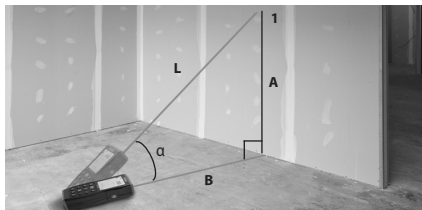
Figur 11 – Indirekte horisontal og vertikal avstand
