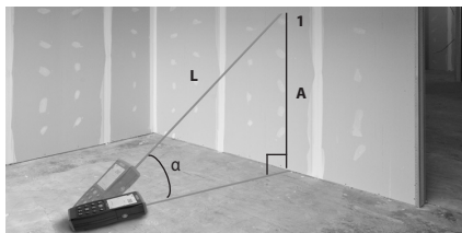
Figur 13 – Indirekte vertikal afstand
