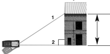
Figure 8 – Mesure indirecte à deux points
