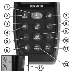
Rys. 3 – Elementy sterujące dalmierza laserowego micro LM-400
