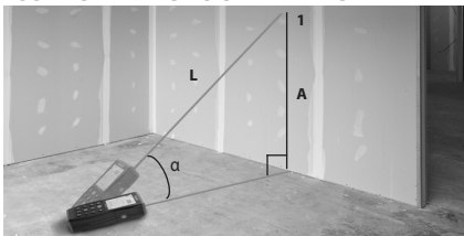
Εικόνα 13 – Έμμεση κατακόρυφη απόσταση
