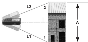
Kuva 14 – Epäsuora pystyettäisyys kahdella pisteellä (kokonaiskorkeus)
