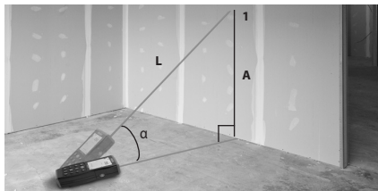
Figuur 13 – Indirecte verticale afstand
