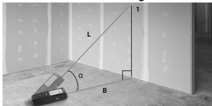
12. ábra – Közvetett vízszintes távolság
