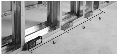
Figura 16 – Medição Piquetagem
