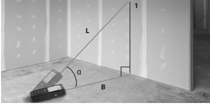
Şekil 12 - Dolaylı Yatay Mesafe
