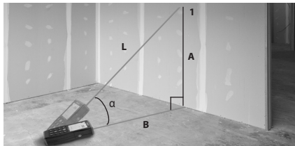
11. ábra – Közvetett vízszintes és függőleges távolság
