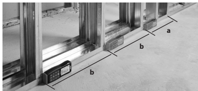
Slika 16 – Mjerenje nadzora
