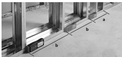
Rys. 16 – Pomiar wytyczania
