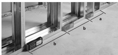
Figuur 16 – Afbakeningsmeting
