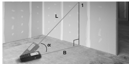
Figure 12 – Mesures horizontales indirectes
