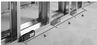
Figura 16 – Măsurare de jalonare
