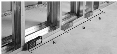
Рисунок 16 – Измерение для разметки
