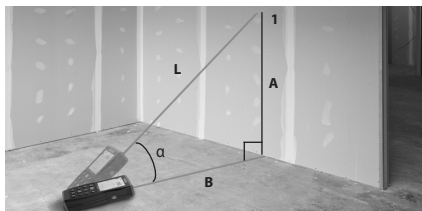
Obrázok 11 – Nepriame meranie horizontálnej a vertikálnej vzdialenosti
