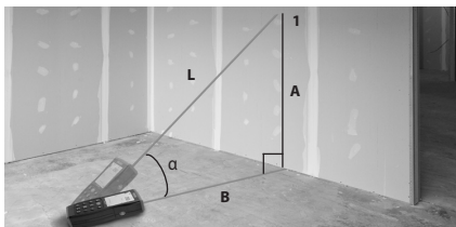
Εικόνα 11 – Έμμεση οριζόντια και κατακόρυφη απόσταση
