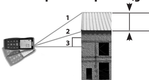
Figuur 10 – Indirecte meting met behulp van drie punten (gedeeltelijke hoogte)
