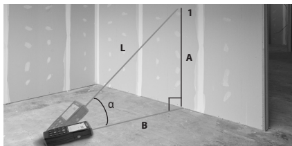
Figura 11 – Distância Indirecta Horizontal e Vertical
