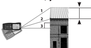
Slika 10 - Neizravno mjerenje uporabom triju točaka (Djelomična visina)
