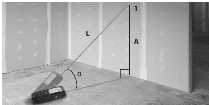
Slika 13 – Indirektna vertikalna razdaljina
