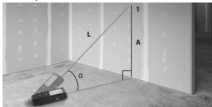
Figura 13 – Distanță verticală indirectă
