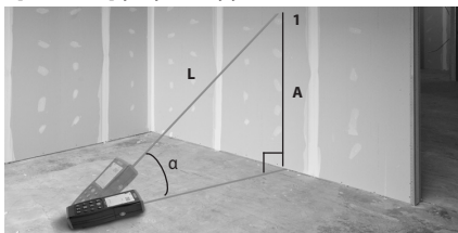
Kuva 13 – Epäsuora pystyetäisyys
