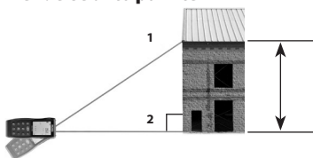
Figur 8 – Indirekte måling ved hjælp af to punkter
