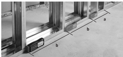
16-сурет — Белгілеу үшін өлшеу
