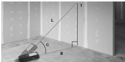
Figur 12 – Indirekte horisontal avstand
