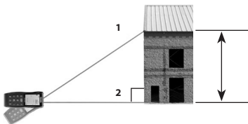
Obrázek 8 – Nepřímé měření s použitím dvou bodů
