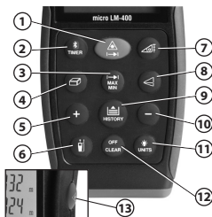
Figur 3 – micro LM-400 Laseravstandsmåler kontrollelementer
