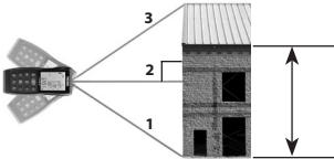
Şekil 9 – Üç Nokta Kullanarak Dolaylı Ölçüm (Toplam Yükseklik)
