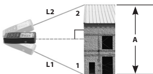
Slika 14 – Indirektna vertikalna razdaljina uz korišćenje dve tačke (celokupna visina)
