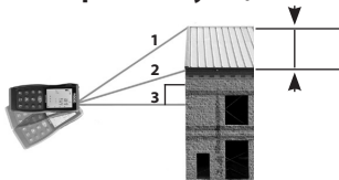
Kuva 10 – Epäsuora mittaus käyttämällä kolmea pistettä (osakorkeus)
