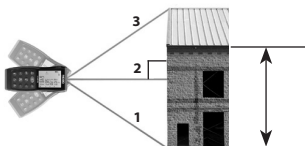
Figura 9 – Medição Indirecta Utilizando Três Pontos (Altura Total)
