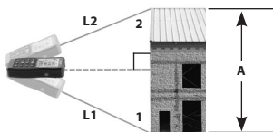
Figur 14 – Indirekte vertikal afstand ved anvendelse af to punkter (samlet højde)
