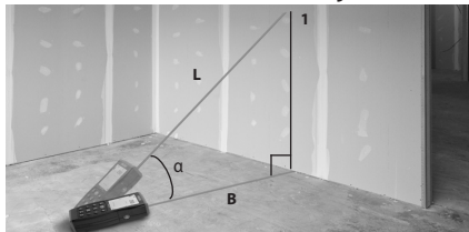
Slika 12 – Indirektna horizontalna razdaljina
