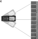
7-сурет — Максимумды және минимумды өлшеу
