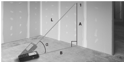
Slika 11 – Neizravna vodoravna i okomita udaljenost
