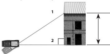
Kuva 8 – Epäsuora mittaus käyttämällä kahta pistettä
