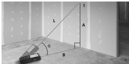
Figuur 11 – Indirecte horizontale en verticale afstand
