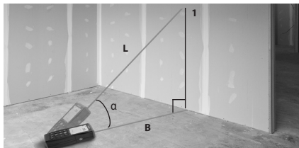
Figura 12 – Distância Horizontal Indirecta
