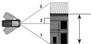
Slika 9 - Neizravno mjerenje uporabom triju točaka (Ukupna visina)
