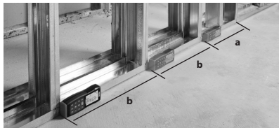
Obrázok 16 – Meranie pomocou dvoch vzdialeností
