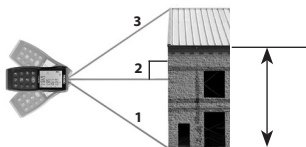
Рисунок 9 –Косвенное измерение между тремя точками (полная высота)
