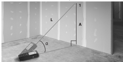
Slika 13 – Neizravna okomita udaljenost
