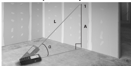
Slika 13 – Posredna navpična razdalja
