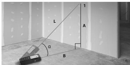
Slika 11 – Posredna meritev vodoravne in navpične razdalje
