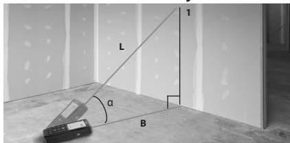
Slika 12 – Posredna vodoravna razdalja
