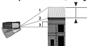
10. ábra – Közvetett mérés három ponttal (részleges magasság)
