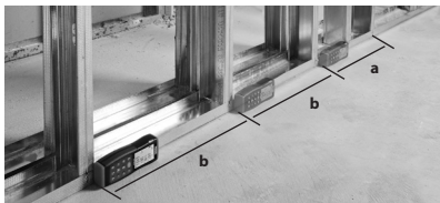
Slika 16 – Meritev za zakoličenje
