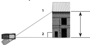
Figur 8 – Indirekt mätning med två punkter
