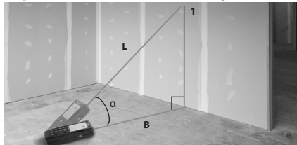
Obrázok 12 – Nepriame meranie horizontálnej vzdialenosti
