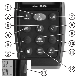
Obrázek 3 – Ovládání laserového dálkoměru micro LM-400
