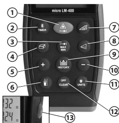
Εικόνα 3 – Πλήκτρα ελέγχου αποστασιόμετρου λέιζερ micro LM-400
