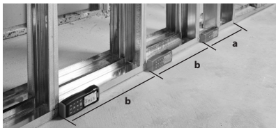
Figur 16 – Utstaket måling
