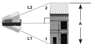
Rys. 14 – Pomiar pośredni odległości pionowej za pomocą dwóch punktów (wysokość całkowita)
