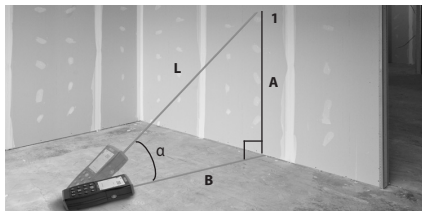
Slika 11 – Indirektna horizontalna i vertikalna razdaljina
