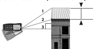
Slika 10 – Posredna meritev s tremi točkami (delna višina)
