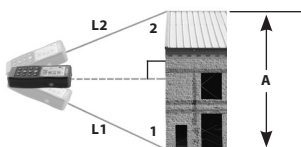
Figura 14 – Distância Vertical Indirecta Utilizando Dois Pontos (Altura Total)
