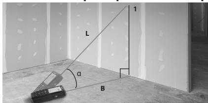
Рисунок 12 – Косвенное измерение расстояния по горизонтали
