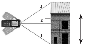
Kuva 9 – Epäsuora mittaus käyttämällä kolmea pistettä (kokonaiskorkeus)
