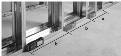
Figur 16 – Utstakningsmätning
