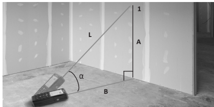
11-сурет — Қашықтықты көлденең және тігінен жанама өлшеу
