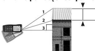
Rys. 10 – Pomiar pośredni za pomocą trzech punktów (wysokość częściowa)
