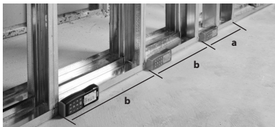
Slika 16 – Merenje razmaka kod postavljanja stubova
