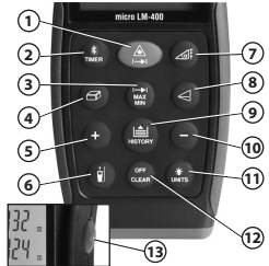
Şekil 3 – micro LM-400 Lazer Mesafe Ölçer Kumandaları
