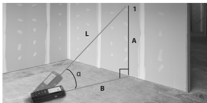
Kuva 11 – Epäsuora vaaka- ja pystyettäisyys
