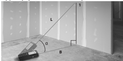
Εικόνα 12 – Έμμεση οριζόντια απόσταση
