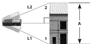
Figur 14 – Indirekte vertikal avstand ved hjelp av to punkter (total høyde)
