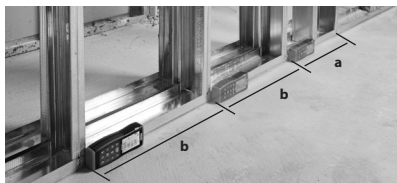
16. ábra – Szakaszmérés
