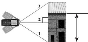
Slika 9 – Posredna meritev s tremi točkami (skupna višina)
