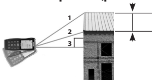
Figur 10 – Indirekt mätning med tre punkter (partiell höjd)
