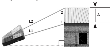
15-сурет — Екі нүкте арасындағы қашықтықты жанама тігінен өлшеу (Ішінара биіктік)
