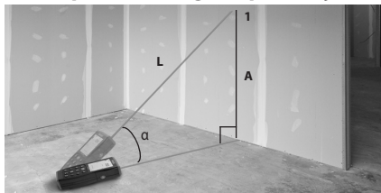
Rys. 13 – Pomiar pośredni odległości pionowej
