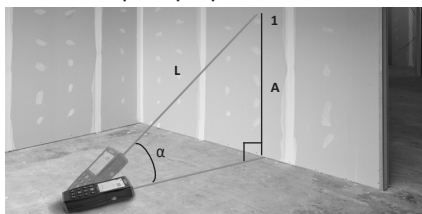
13-сурет — Жанама тік қашықтық
