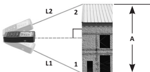
14-сурет — Екі нүкте арасындағы қашықтықты жанама тігінен өлшеу (Жалпы биіктік)
