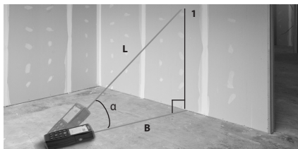
Figuur 12 – Indirecte horizontale afstand
