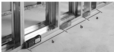
Figur 16 – Afmærkningsmåling
