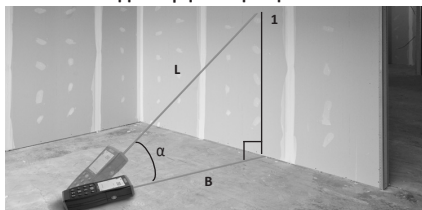
12-сурет — Жанама көлденең қашықтық
