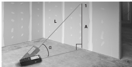
Figur 13 – Indirekt lodrät sträcka
