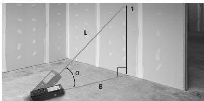
Figur 12 – Indirekte horisontal afstand
