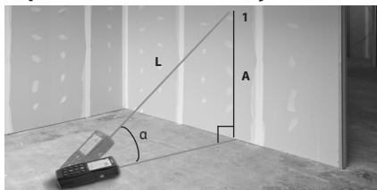
Obrázok 13 – Nepriame meranie vertikálnej vzdialenosti
