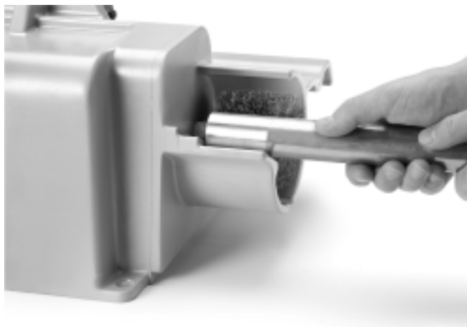
図7 外面研磨
