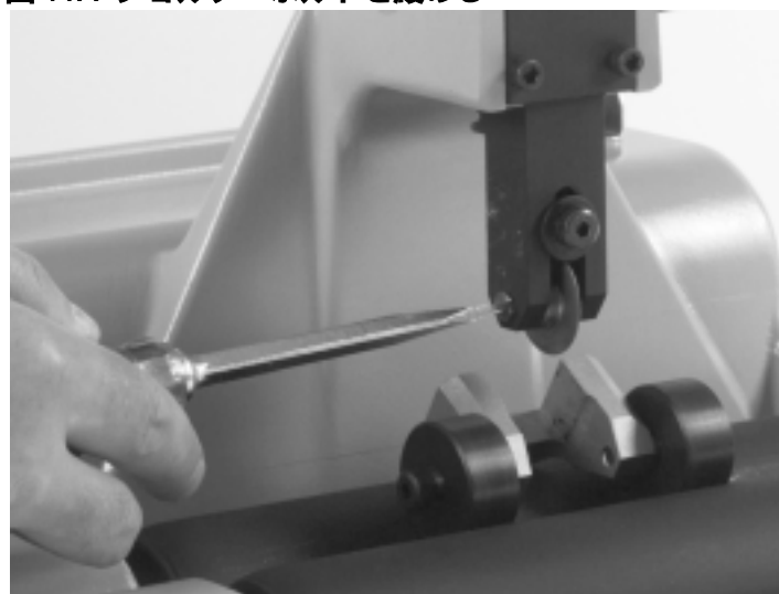
図 11A ショルダーボルトを緩める
