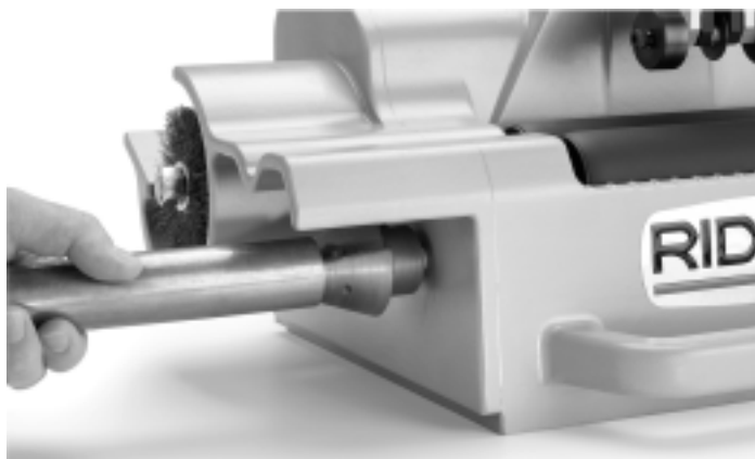
図8 内面リーマ
