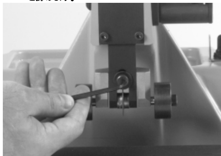
図 11A ショルダーボルトを緩める
