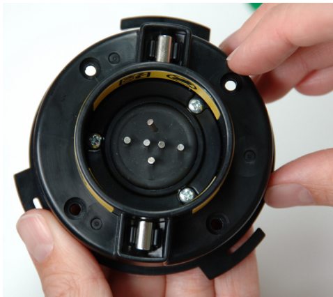
Afbeelding 6 – Gebroken contactpen
