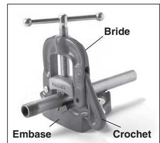
B. Etau d'établi à bride
