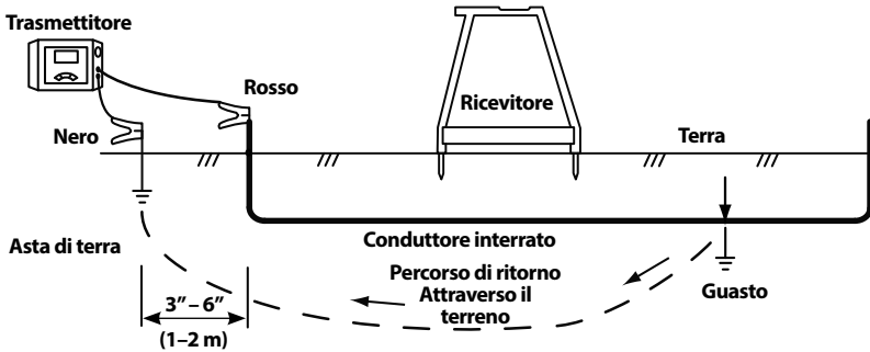
Figura 8 – Connessioni del trasmettitore per l'individuazione dei guasti
