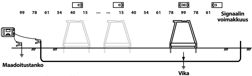
Kuva 11 – Signaalinvoimakkuus
