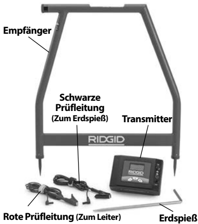
Abbildung 1 – Dreiecksrahmen-Fehlersuchgerät
