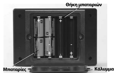
Εικόνα 6 – Αλλαγή μπαταριών (πομπός)
