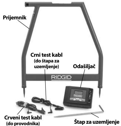
Slika 1 – Lokator oštećenja sa A-ramom
