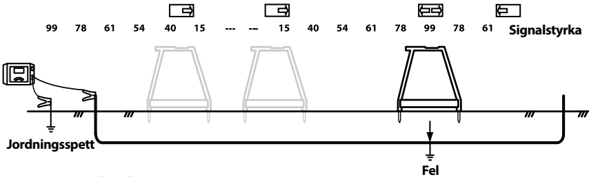
Figur 11 – signalstyrka
