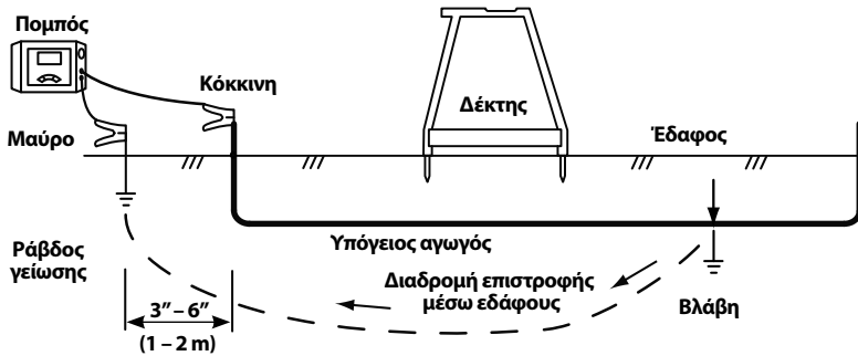
Εικόνα 8 – Συνδέσεις πομπού για τον εντοπισμό βλαβών
