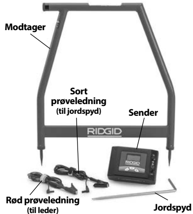
Figur 1 – Fejlsøger med A-formet ramme Sender
