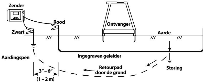
Figuur 8 - Zenderaansluitingen voor het opsporen van storingen
