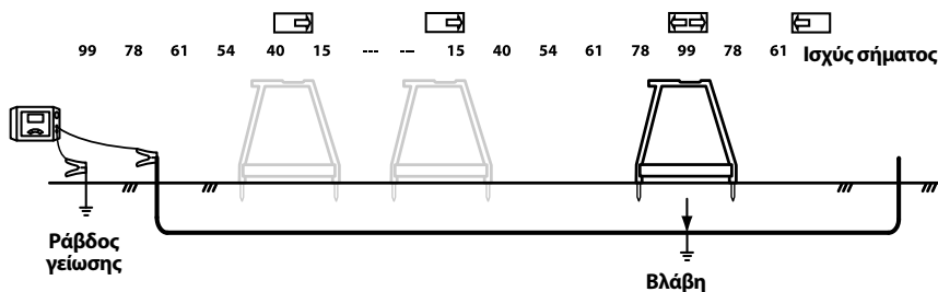
Εικόνα 11 - Ισχύς σήματος
