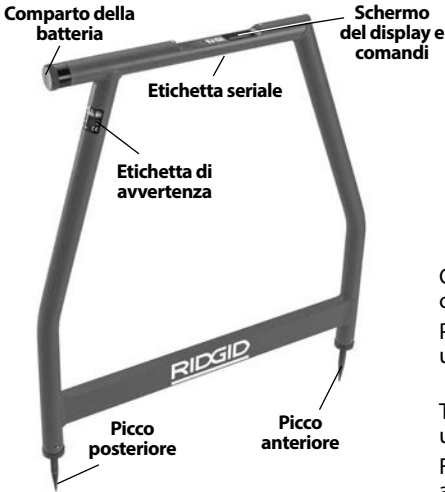
Figura 4 – Ricevitore A-Frame
