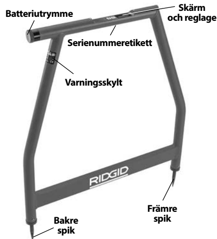
Figur 4 – Tvåbensbockmottagare
