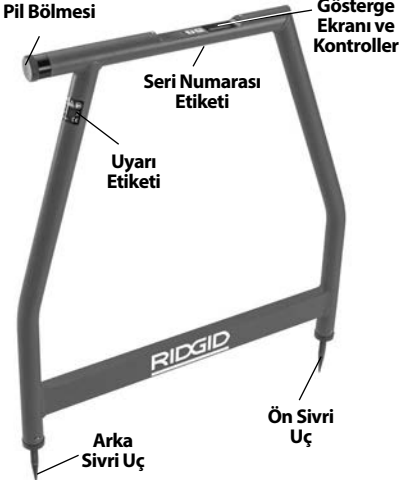
Şekil 4 – A Frame Alicısı
