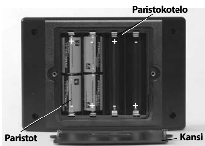
Kuva 6 – Paristojen vaihtaminen (lähetin)
