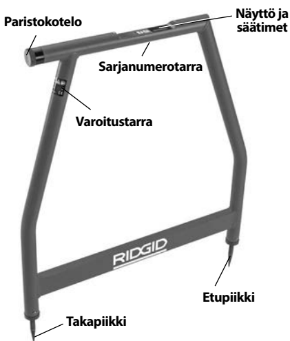
Kuva 4 – A-runkoinen vastaanotin
