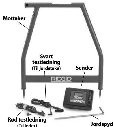
Figur 1 – A-Frame Feillokaliseringsverktøy
