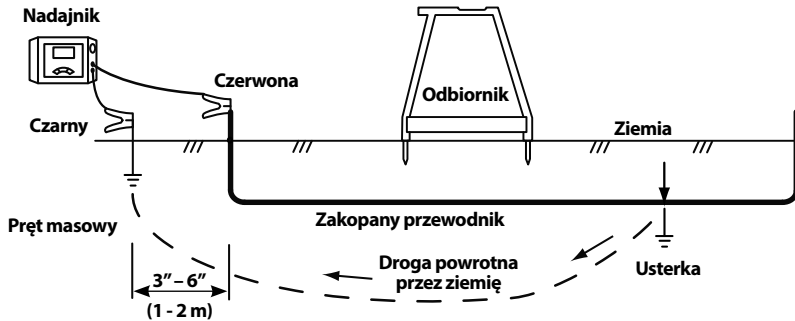
Rysunek 8 - Podłączenia nadajnika do znajdowania usterek
