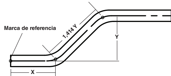
B – Tubo doblado con marcas
