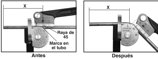
Figura 5 – Alineamiento para curvar en 45°
