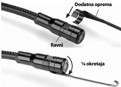
Slika 8 - Montaža dodatne opreme
