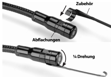
Abbildung 8 - Einbau von Zubehöerteilen
