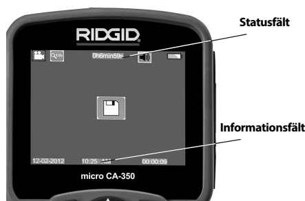
Figur 12 – Realtidsskärbild
