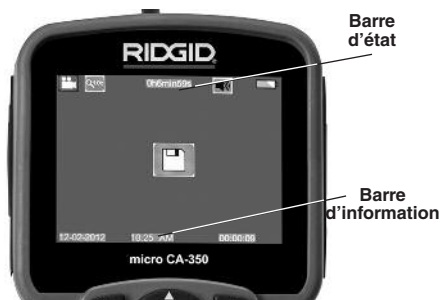
Figure 12 – Ecran vidéo
