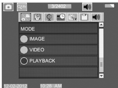
Rys. 17 - Ekran ustawień
