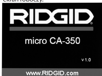
Rys. 11 - Ekran powitalny
