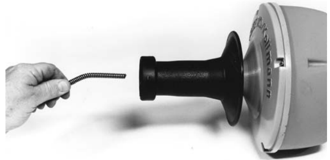
Figure 11 – Insertion de l'embout de câble dans le tambour
