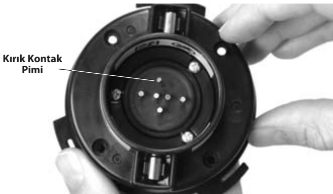
Şekil 12 – Kırık Kontak Pimi
