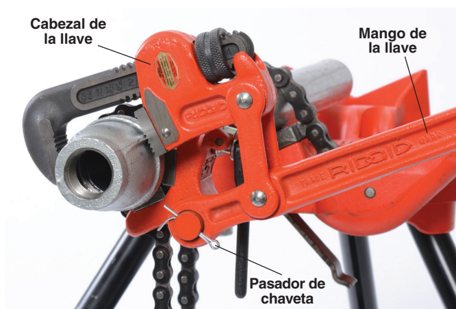
Figura 6 B – Fijación del mango al muñón
