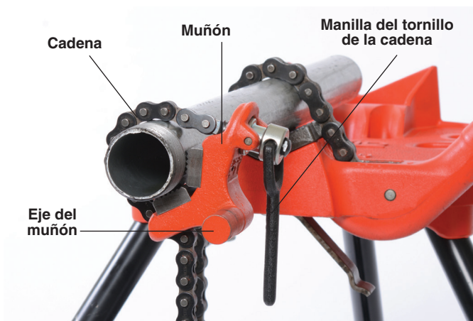
Figura 6 A – Montaje del muñón de la llave de palanca compuesta sobre el tubo
