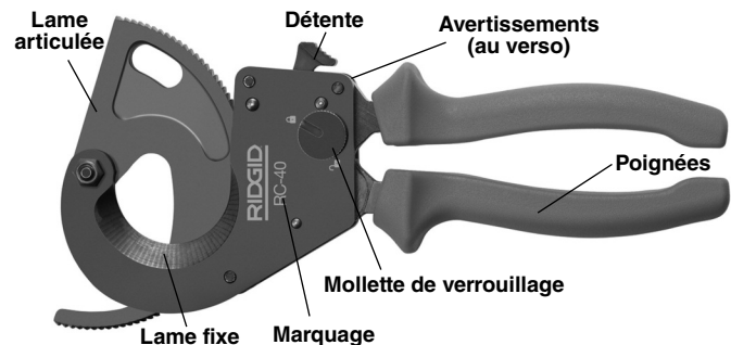
Figure 1 – Coupe-câbles à crémaillère (modèle RC-40 affiché)
